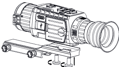
Рис. 2-5. Установка устройства и затягивание винтов
