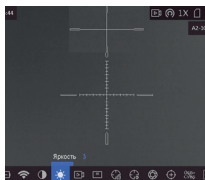
Рис. 2-7. Интерфейс меню
